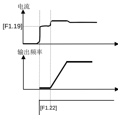
图 6-9 启动预励磁输出
