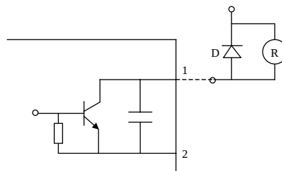
图 6-13 OC 输出端子的内部线路
