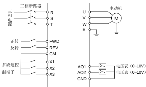
图 9-3 基本接线图
