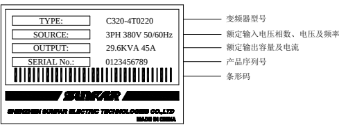
图-1 变频器铭牌数据
