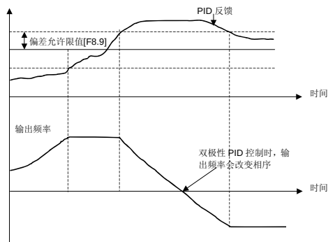
图 6-31 双极性 PID 控制方式
