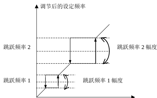
图 6-27 跳跃频率输出
