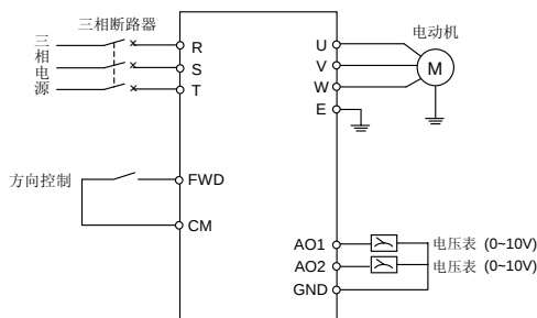
图 9-1 基本接线图
