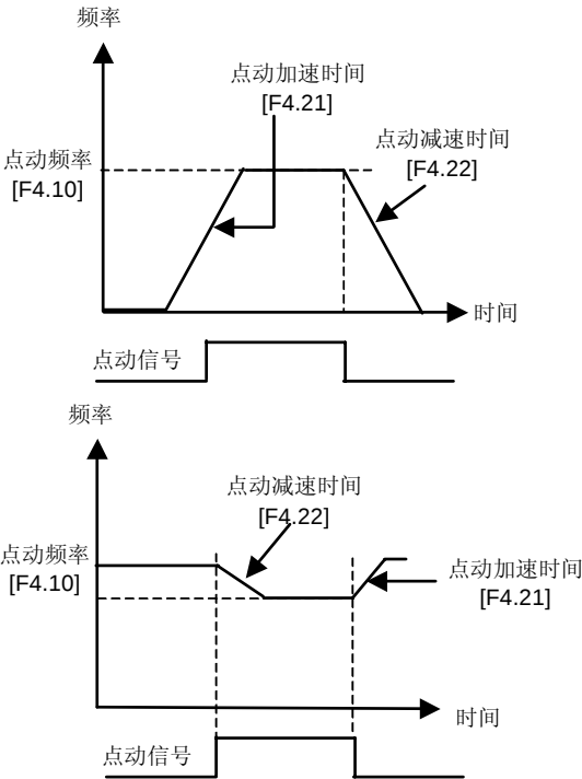
图 6-19 点动运行
