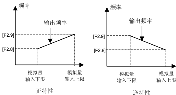
图 6-10 模拟输入与设定频率对应图示
