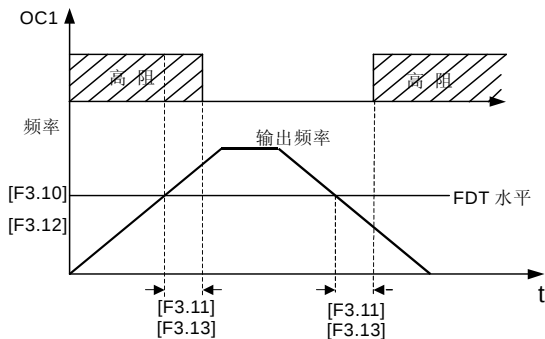
图 6-15 频率水平检测 (FDT)
