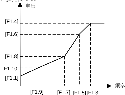
图 6-6 V/F 自定义曲线设定
