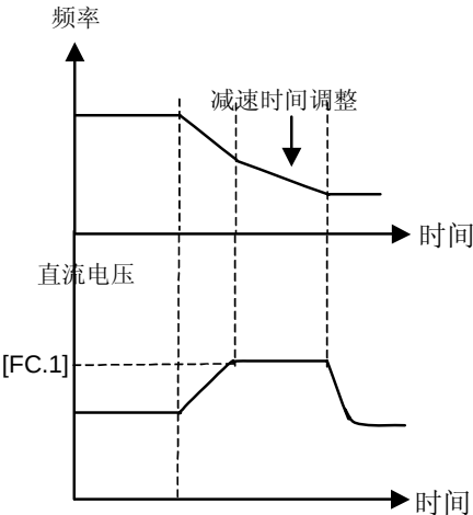
图 6-35 减速中的电压失速保护
