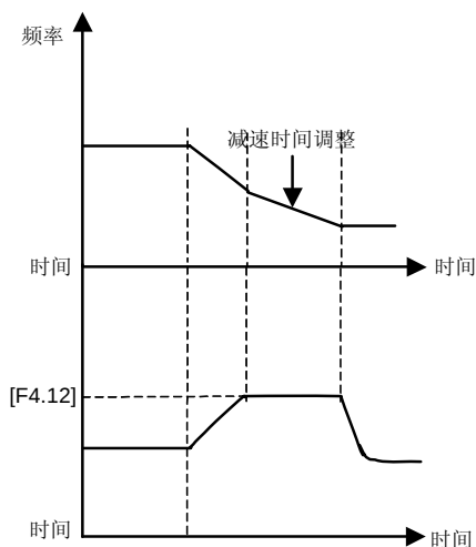
图 6-20 加速力矩与制动力矩示意图
