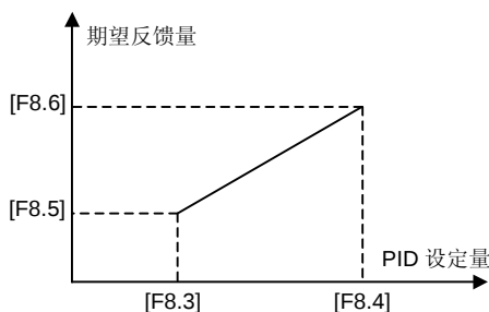
图 6-32 PID 给定量与反馈量的关系
