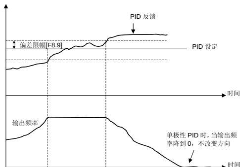
图 6-30 单极性 PID 控制方式
