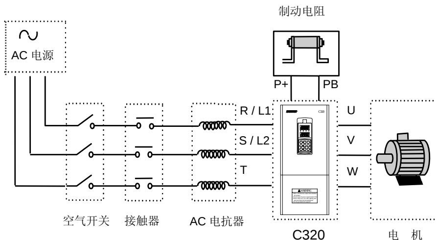
图 3-2 变频器的配线图
