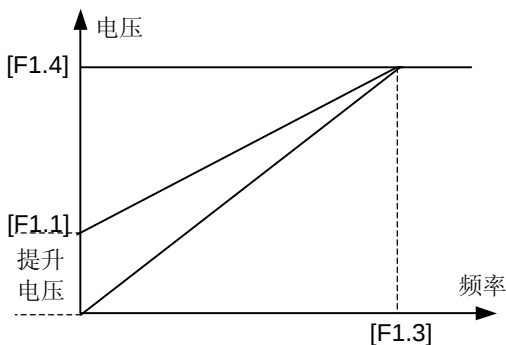
(2) 恒转矩曲线转矩提升示意图
