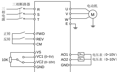
图 9-2 基本接线图
