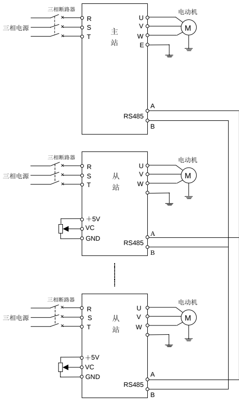
图 9-5 基本接线图
