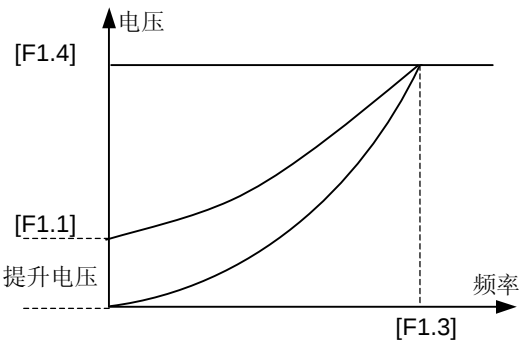
(1) 降转矩曲线转矩提升示意图
