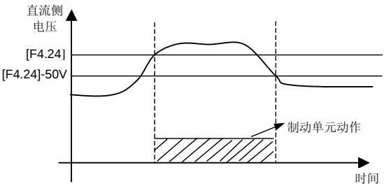
图 6-23 能耗制动
