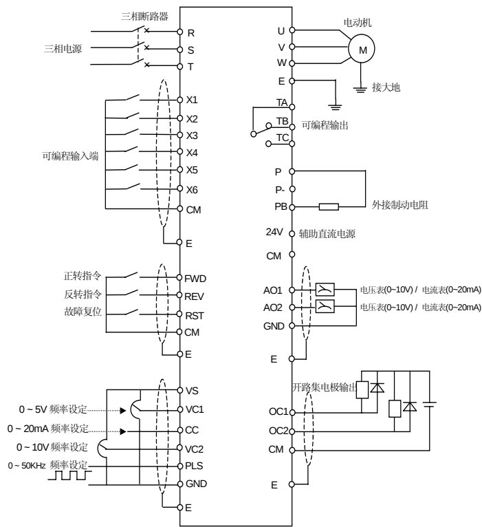
图 3-3 C320 系列变频器基本接线图
