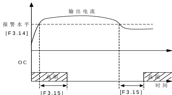
图 6-16 过载报警
