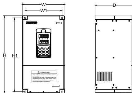
图 2-4-B 变频器安装尺寸
