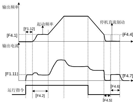
图 6-7 启动与停机过程
