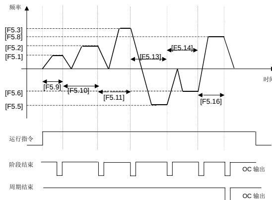
图 6-24 单循环停机模式
