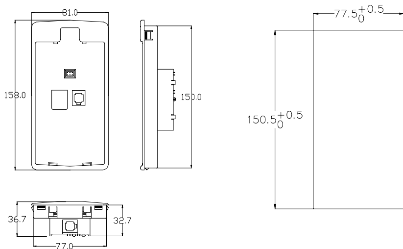
图-B 操作面板底座安装开孔尺寸
