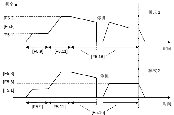
图 6-24 PLC 断点恢复
