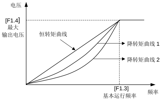
图 6-4 V/F 曲线
