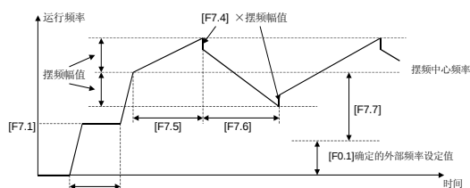
6-28 摆频运行过程
