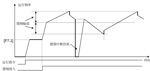
6-29 断点记忆恢复（条件有效方式）
