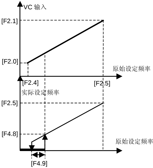
图 6-18 频率输出过零点曲线
