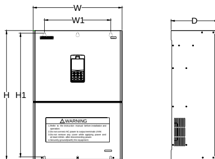
图 2-4-C 变频器安装尺寸
