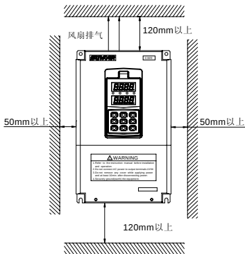
图 2-1-A 安装的间隔距离
