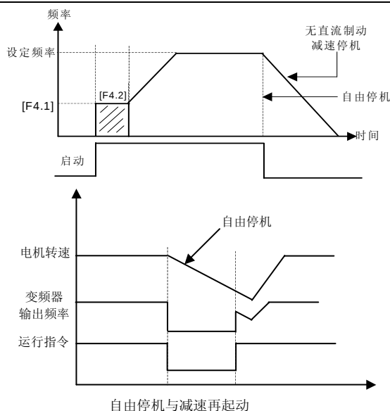
图 6-17 启动与停机频率输出曲线
